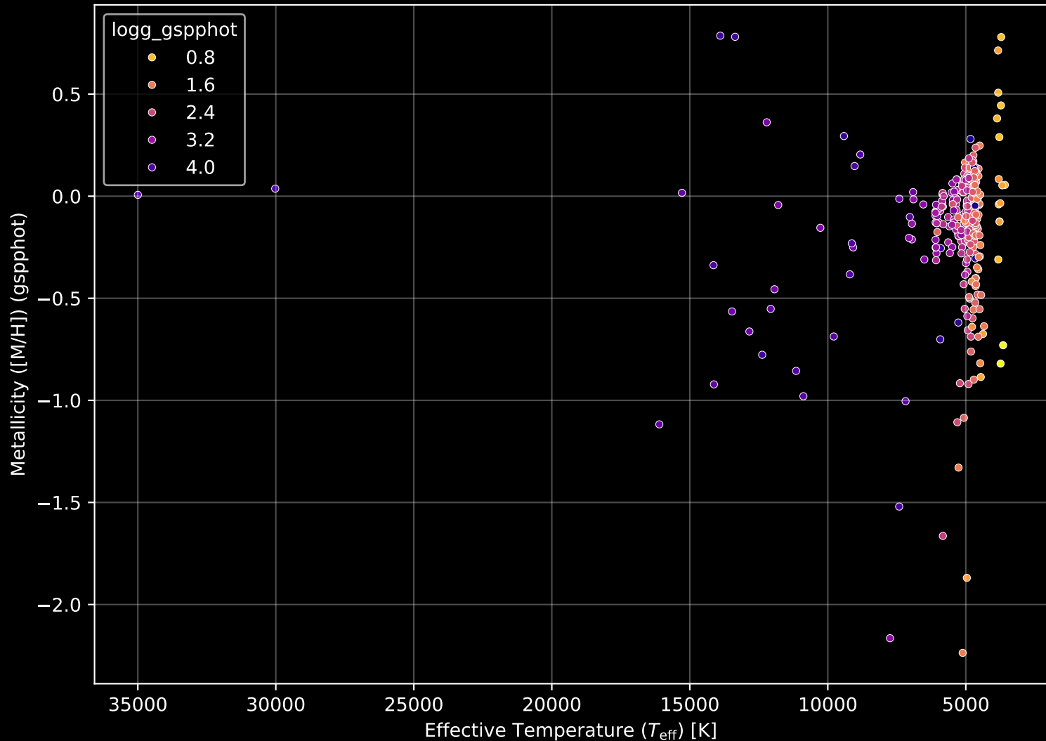
APOGEE DR17 Field: [161+00] Stellar Population Parameters (n= 304)
